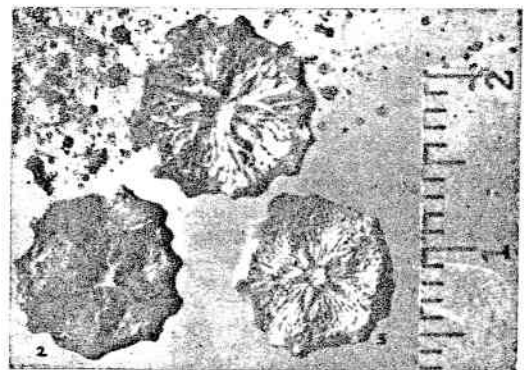
Cara ventral de la pieza centro dorsal del Salanocrinus astrei BATALLER.
