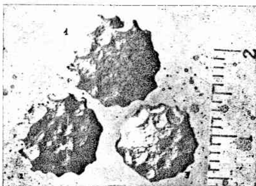
Cara dorsal de los mismos ejemplares.
