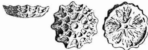
Dibujo, no muy afortunado, del Solanocrinus astrei BATALLER, que aparece en la publicación del Dr. Bataller, y a cuyos defectos alude en la diagnosis.
